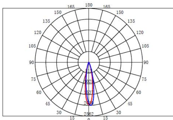
配光曲线
