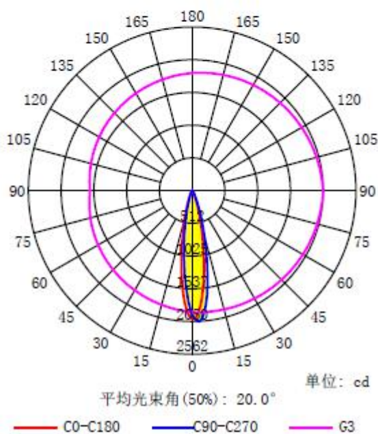
配光曲线
